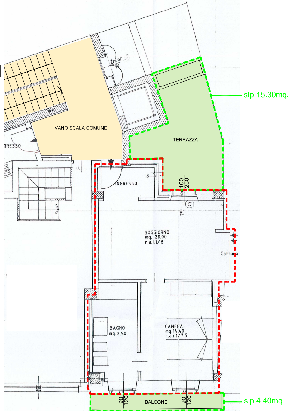
PIANTA P. PRIMO 1:100
